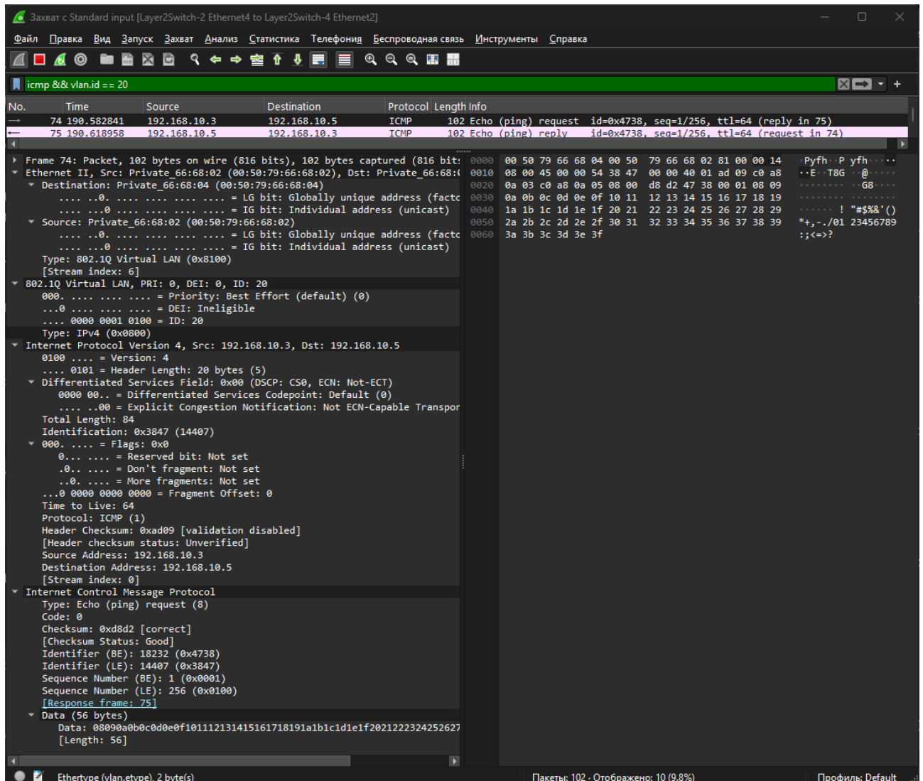
Рисунок 3 — Перехват ICMP-пакета VLAN20 с тегом IEEE 802.1Q
