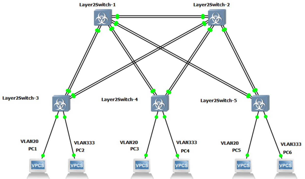
Рисунок 1 — Физическая топология сети для настройки VLAN
