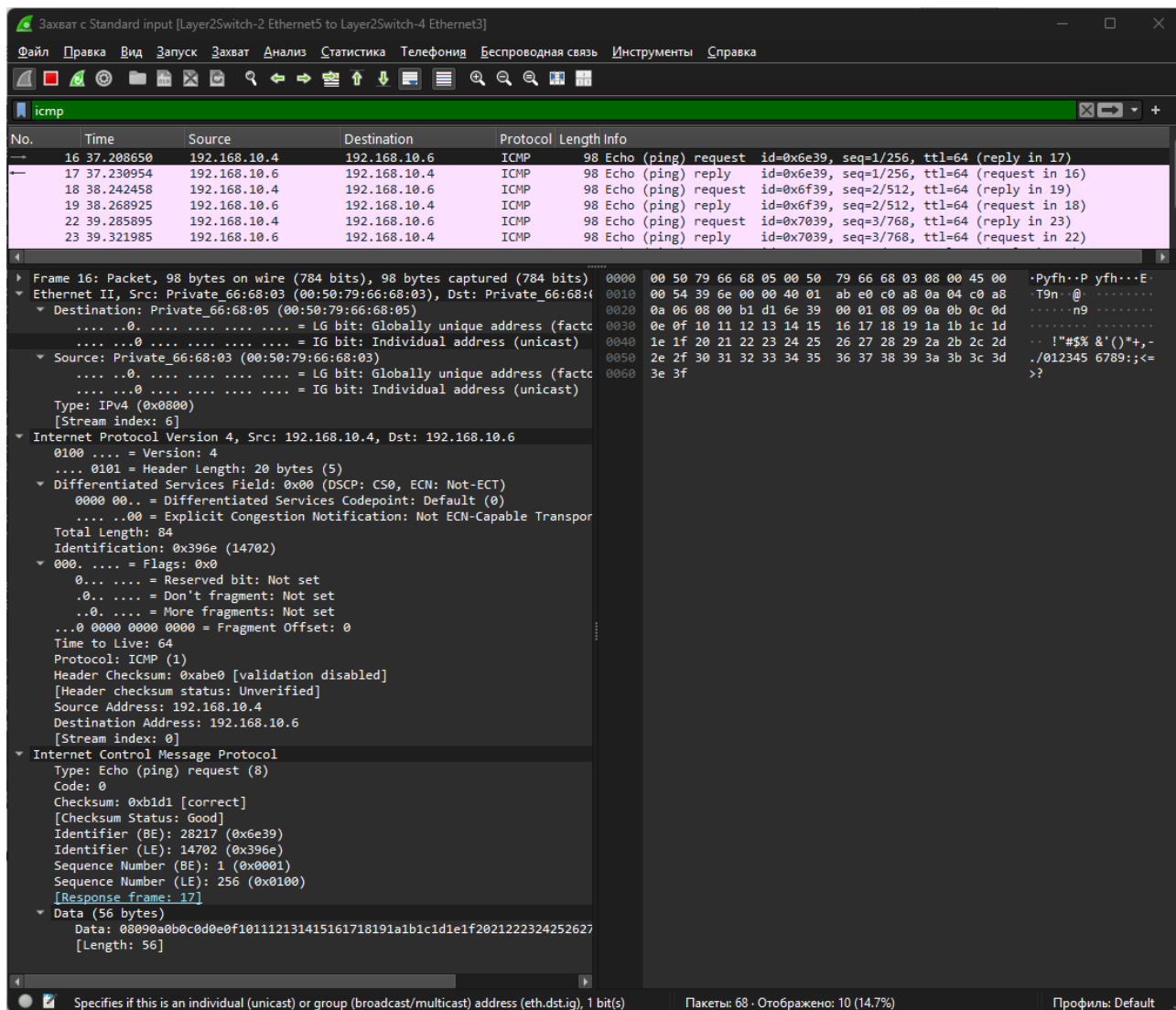
Рисунок 4 — Перехват ICMP-пакета Native VLAN333 без тега IEEE 802.1Q
